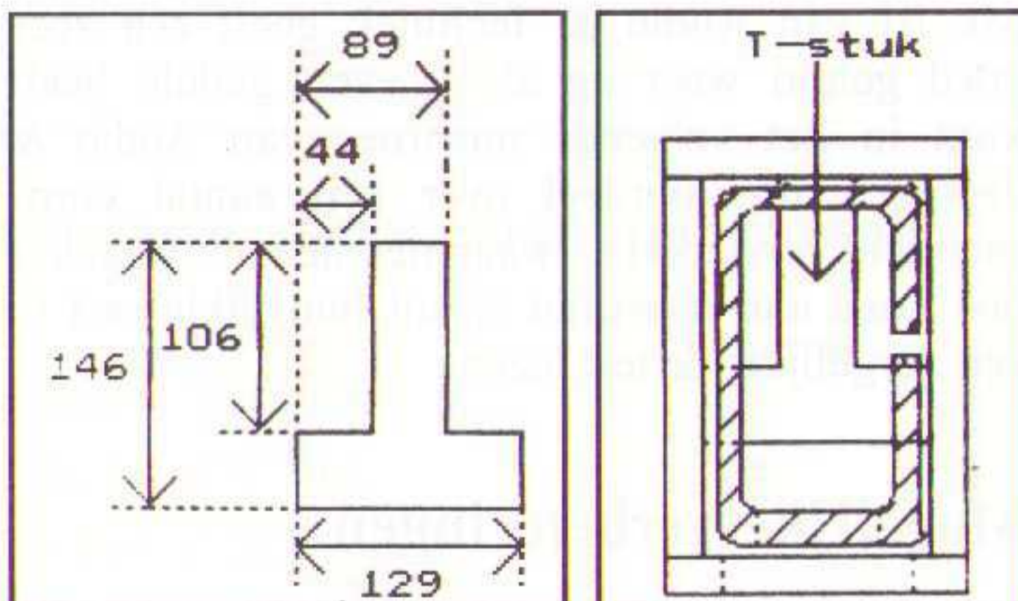
Figuur 6. Het achter de basunit aan te brengen T-stuk.
